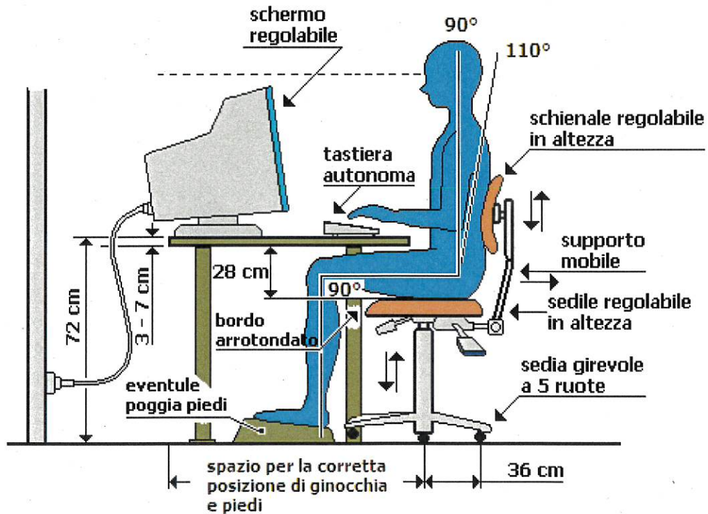
Allegato 2 – Schema "disposizione della postazione di lavoro"
